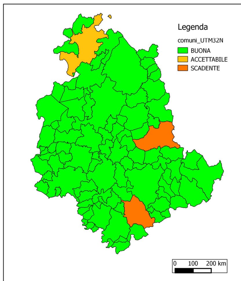
Figura 7.1: Lo stato della qualità dell'aria per l'anno 2013 per \text{PM}_{10} . Le valutazioni ottenute con misure integrate al modello sono rappresentate a scala comunale anche quando le criticità (qualità accettabile e/o scadente) interessano un'area sub comunale.
