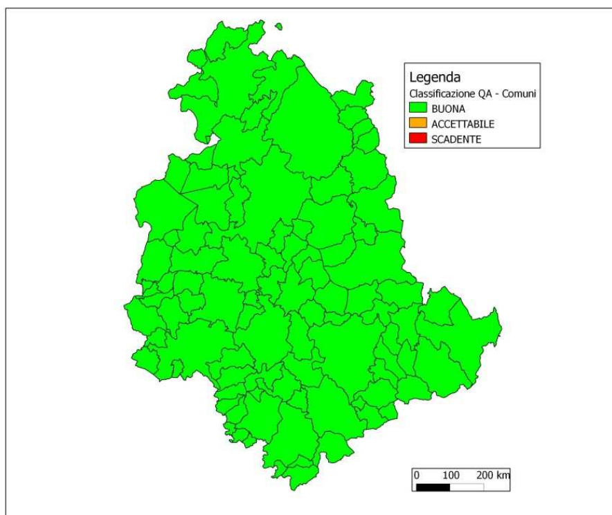
Figura 7.5: Lo stato della qualità dell'aria per l'anno 2013 per SO 2 . Le valutazioni ottenute con misure integrate a modelli sono rappresentate a scala comunale anche quando le criticità (qualità accettabile e/o scadente) interessano un'area sub comunale.
