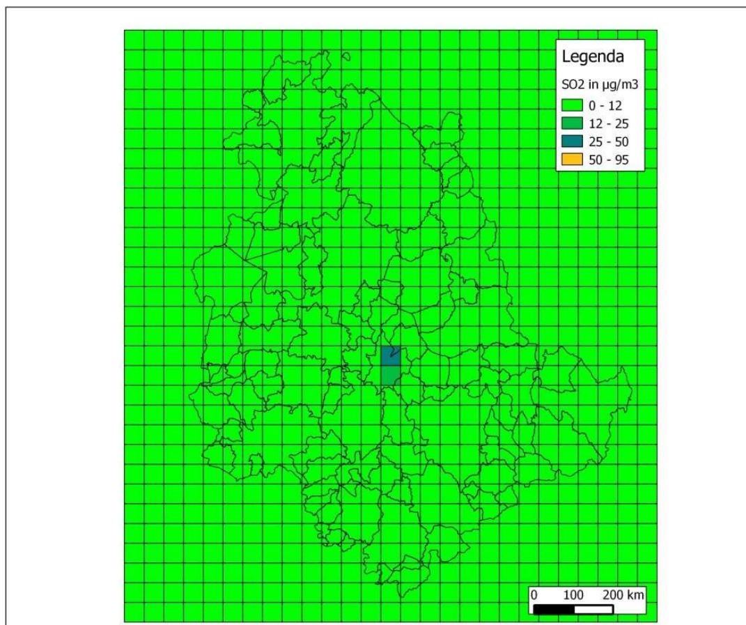
Figura 6.7: Concentrazione media annua di SO 2
