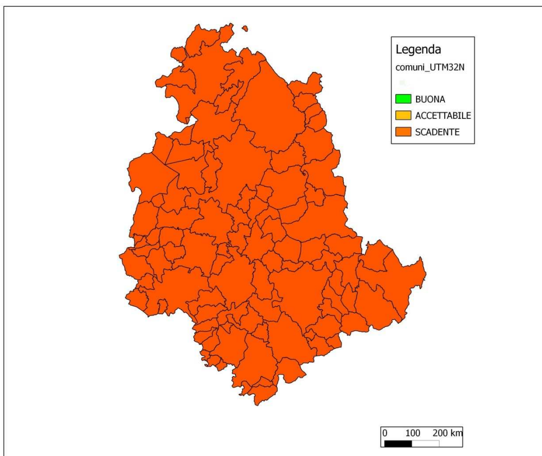
Figura 7.9: Lo stato della qualità dell'aria per l'anno 2013 per Ozono. Le valutazioni ottenute con misure e modellistica è fatta rispetto all'obiettivo lungo termine in quanto tale indice ha valenza annuale
