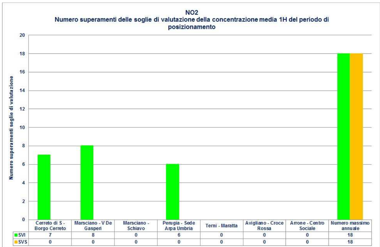
Figura 5.5: Numero superamenti della concentrazione media 1h per NO 2 riferita al periodo di presenza della stazione mobile presso il sito - confronto con le soglie di valutazione
