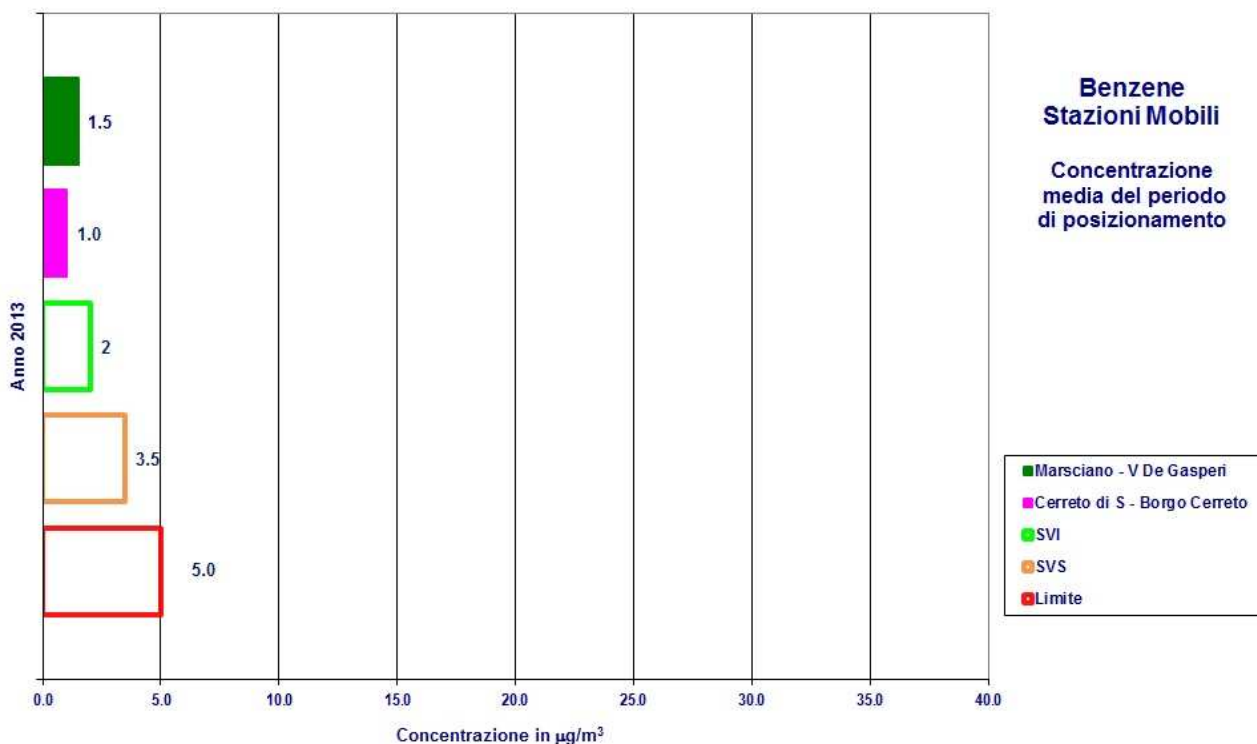
Figura 5.9: Concentrazione media per Benzene riferita al periodo di presenza della stazione mobile presso il sito - confronto con limite e soglie di valutazione
