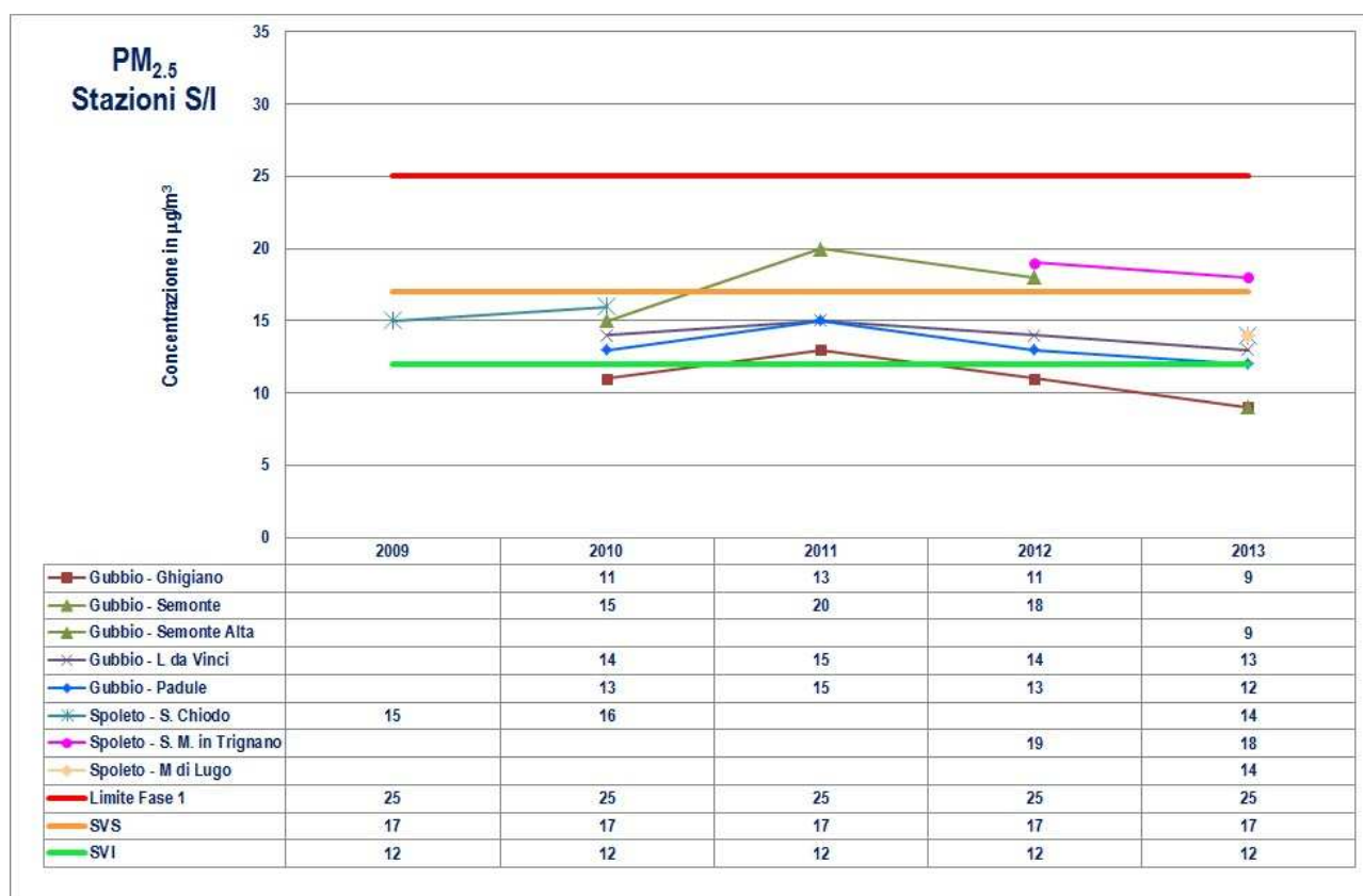
Figura A1.3: Trend 2009 - 2013 concentrazione media annua del PM 2.5 divisi per tipologia di stazione (U/T-I= Urbana da Traffico e Industriale, U/F = Urbana di Fondo, S/F = Suburbana di Fondo, R/F = Rurale di Fondo, S/I = Suburbana Industriale)
