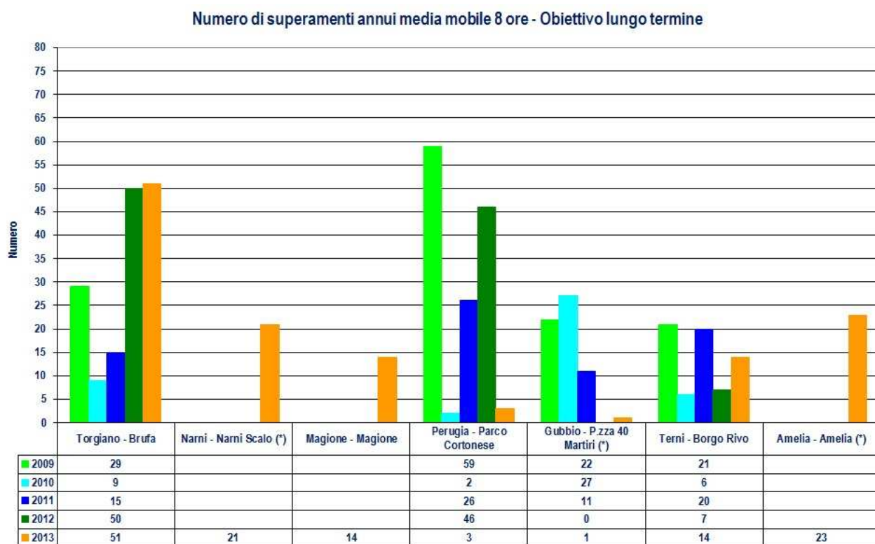
Figura A1.19: Trend 2009 - 2013 del numero di superamenti annui della concentrazione media mobile 8 ore di O 3 - Obiettivo lungo termine
