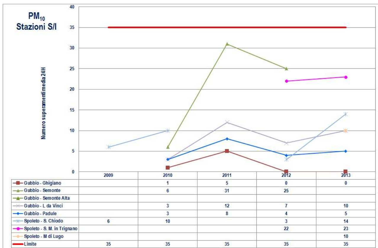
Figura A1.2: Trend 2009 - 2013 numero superamenti concentrazione media 24h del PM 10 divisi per tipologia di stazione (U /T-I= Urbana da Traffico e Industriale, U/F = Urbana di Fondo, S/F = Suburbana di Fondo, R/F = Rurale di Fondo, S/I = Suburbana Industriale)
