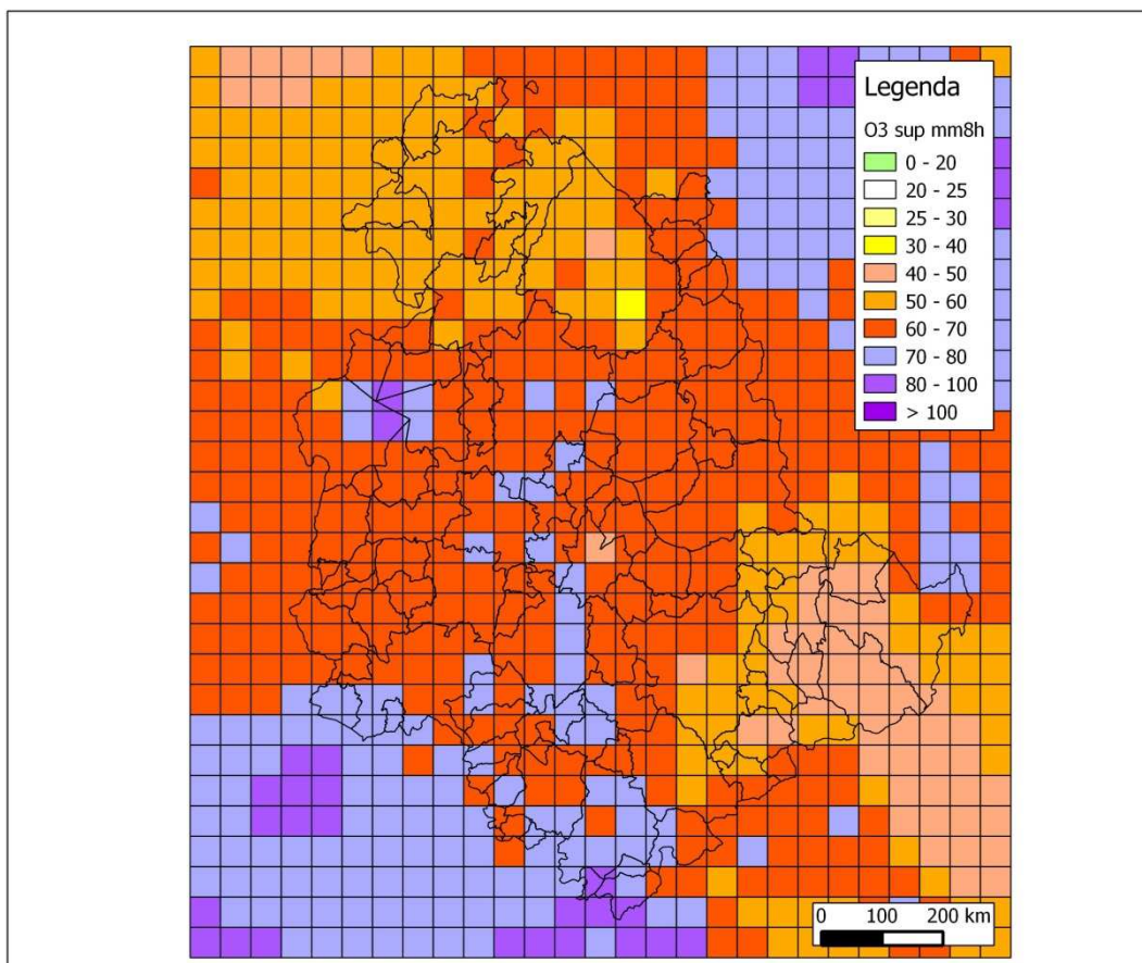
Figura 6.10: Obiettivo lungo termine numero dei giorni di superamento della soglia di 120 \mu\text{g}/\text{m}^3 quale media massima giornaliera calcolata su 8 ore
